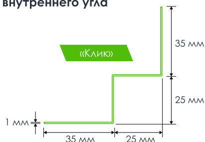
Профиль внутреннего угла
